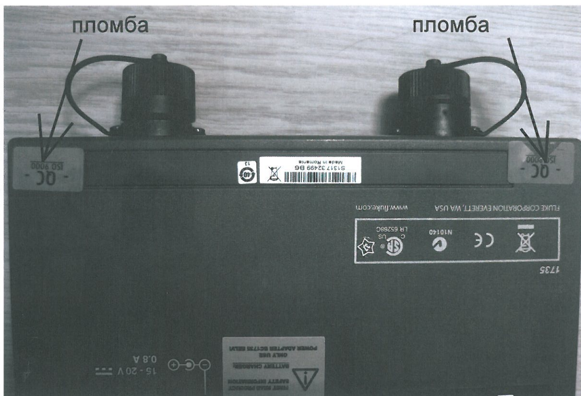
Рисунок 2. Схема пломбирования регистраторов модели Fluke 1735.
